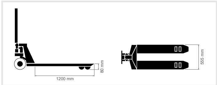
Dimensões principais
