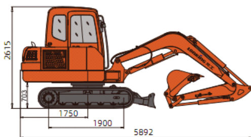
Dimensões principais
