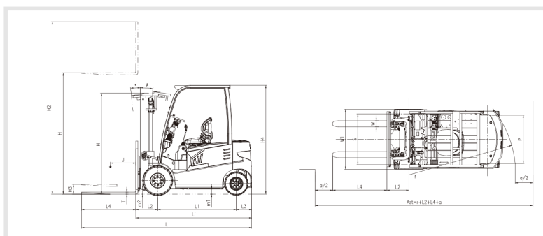
Dimensões principais
